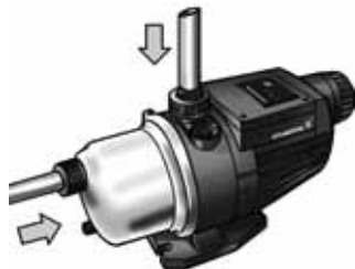
Рис. 5 Монтаж всасывающей и напорной линий к насосной установке MQ
